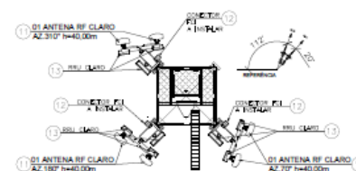
PLANTA DE NÍVEL
