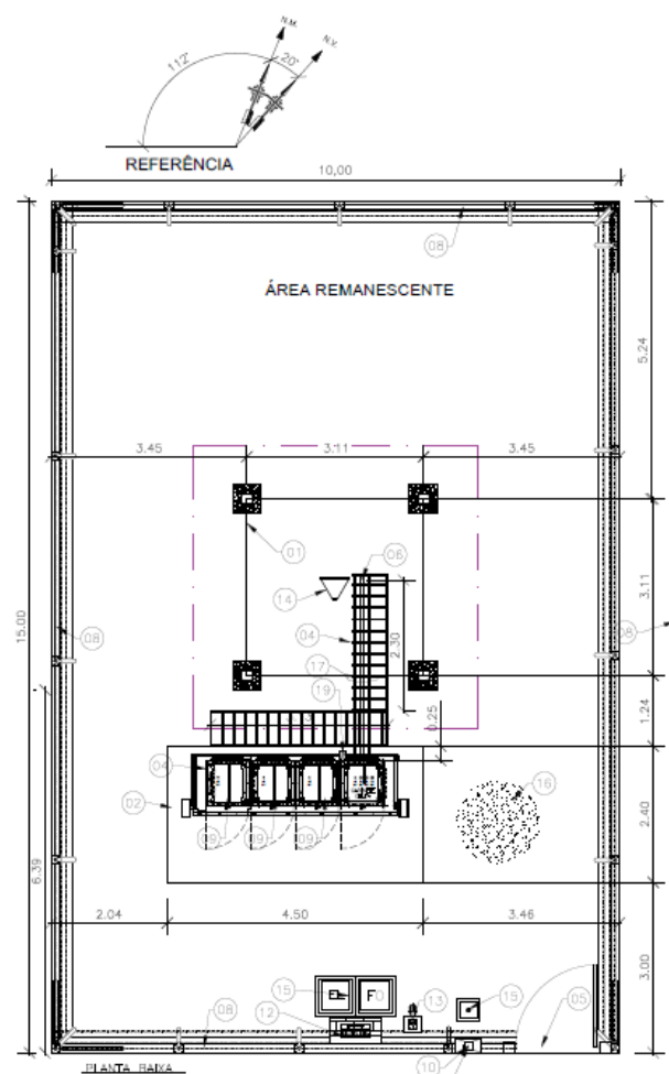
PLANTA BAIXA
