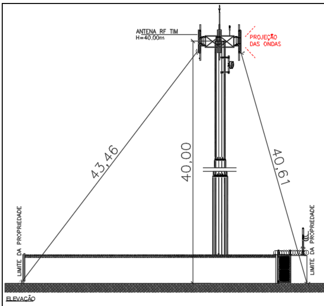
Figura 08 – Representação gráfica da situação em escala, com as cotas e distâncias do ponto de emissão das ondas eletromagnéticas em relação às edificações imediatamente vizinhas.
